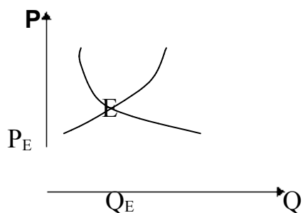
Рис. 2.1. Ціна рівноваги
