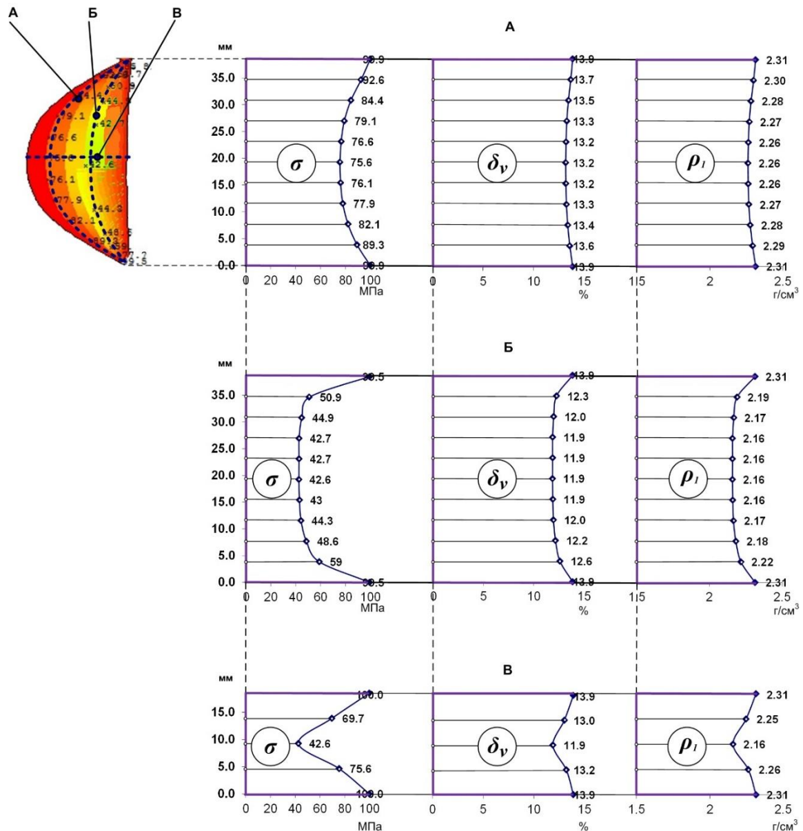
Рисунок 5 – Розподіл в брикеті напружень ( \sigma ), пружної післядії ( \delta_v ) та щільності ( \rho_1 ), конфігурація формуючих елементів зубчато-жолобчата, матеріал – марганцевий концентрат (фр. -3 мм)
