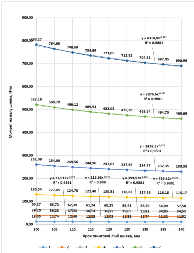
Рисунок 13 – Зв'язок величини моменту на валу шнека з кроком гвинтової лінії висота стовпа шихти над входом в шнек: 1 – 5 мм; 2 – 15 мм; 3 – 25 мм; 4 – 50 мм; 5 – 100 мм; 6 – 200 мм; 7 – 300 мм; матеріал – торф
