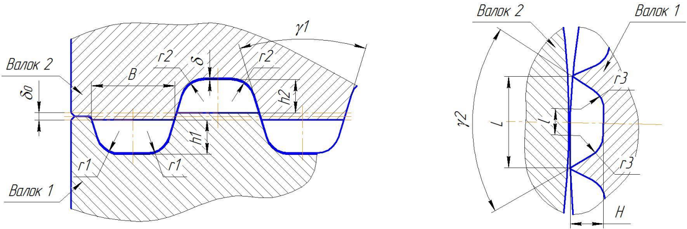
Рисунок 6 – Новий тип формуючих елементів
