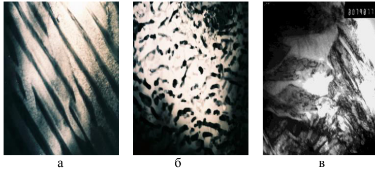
Рис. 1. Фрагменти продуктів розпаду аустеніту в чавуні у литому стані, отримані методом просвітлювальної електронної мікроскопії: а – \times 37000 ; б – \times 30000 ; в – \times 30000
