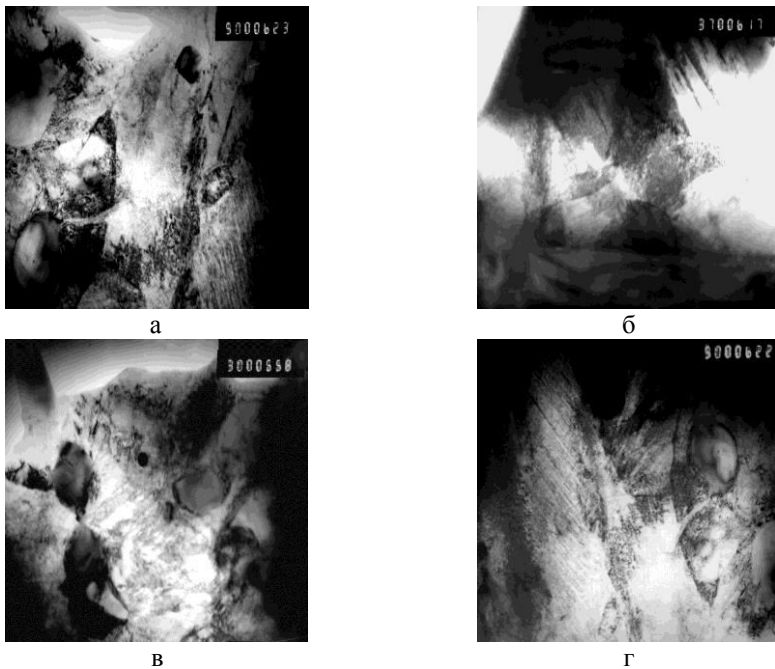
Рис. 2. Фрагменти продуктів розпаду аустеніту, отримані методом просвітлювальної електронної мікроскопії: а – \times 50000 ; б – \times 37000 ; в – \times 30000 ; г – \times 50000
