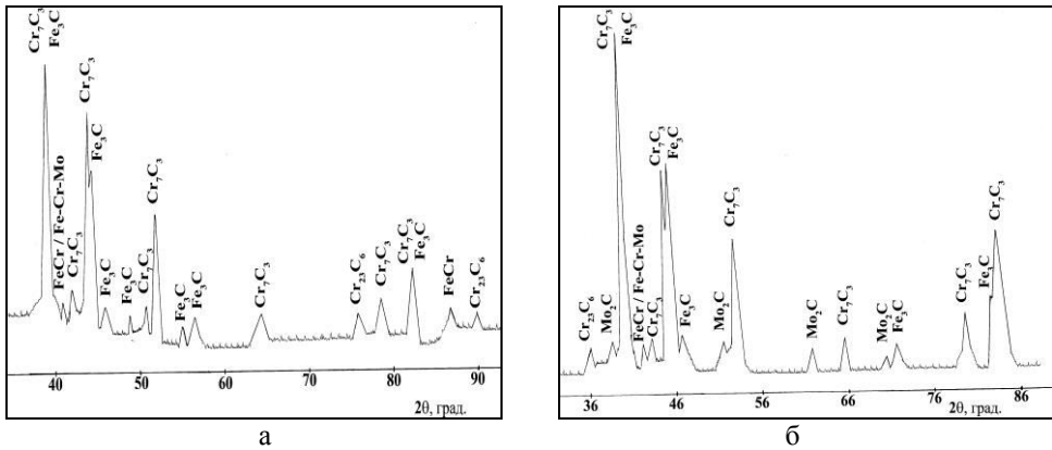
Рис. 4. Ділянки дифрактограм карбідного осаду зразків чавуну з вмістом хрому 21,0-21,4% у литому стані після повторного нагріву при: а – T=680^{\circ}\text{C} ; б – T=480^{\circ}\text{C}
