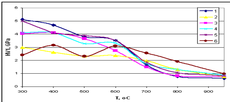
Рис. 11 Температурна залежність гарячої міцності зразків чавуну типу 28X32НЗФ та хромонікелевого сплаву «нікорим»: 1 – литий стан; 2 – T_{\text{ауст}}=950^{\circ}\text{C} , \tau_{\text{ауст}}=1\text{год} ; T_{\text{ізот}}=350^{\circ}\text{C} , \tau_{\text{ізот}}=3\text{год} ; 3 – T_{\text{ауст}}=950^{\circ}\text{C} , \tau_{\text{ауст}}=1\text{год} ; T_{\text{ізот}}=350^{\circ}\text{C} , \tau_{\text{ізот}}=5\text{год} ; 4 – T_{\text{ауст}}=1050^{\circ}\text{C} , \tau_{\text{ауст}}=1\text{год} ; T_{\text{ізот}}=350^{\circ}\text{C} , \tau_{\text{ізот}}=3\text{год} ; 5 – T_{\text{ауст}}=1050^{\circ}\text{C} , \tau_{\text{ауст}}=1\text{год} ; T_{\text{ізот}}=350^{\circ}\text{C} , \tau_{\text{ізот}}=5\text{год} ; 6 – «нікорим» у литому стані.
