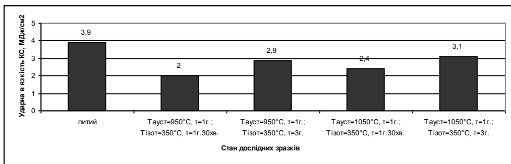
Рис.8 Залежність ударної в'язкості дослідного чавуну від температури аустенізації та часу витримки при температурі 350°C
