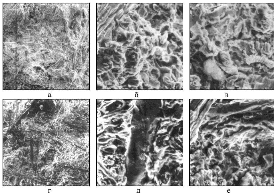
Рис. 10 Мікрофрактограми зламів дослідного чавуну після термічної обробки за режимом: а - в – T_{\text{ауст}}=1050^{\circ}\text{C} , \tau_{\text{ауст}}=1\text{г.} , T_{\text{ізот}}=350^{\circ}\text{C} , \tau_{\text{ізот}}=1\text{г.30хв.} ; г - е – T_{\text{ауст}}=1050^{\circ}\text{C} , \tau_{\text{ауст}}=1\text{г.} , T_{\text{ізот}}=350^{\circ}\text{C} , \tau_{\text{ізот}}=3\text{г.} , (а, г – х100, б, в, д, е – х1000), РЕМ
