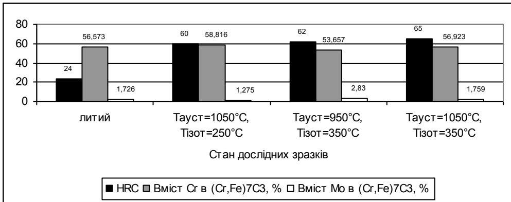
Рис. 3. Вплив кількості залишкового аустеніту та ступеню його легованості (а), вмісту хрому та молібдену у евтектичному карбіді (Cr, Fe)_7C_3 (б) на твердість високохромистого чавуну у литому та термообробленому стані
