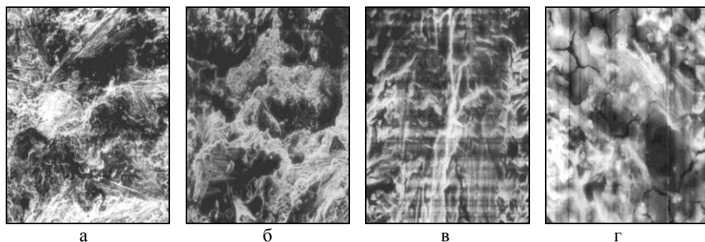
Рис. 9 Мікрофрактограми зламів чавуну у литому стані (а-б – х100, в-г – х1000), РЕМ
