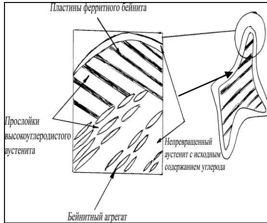
Рис. 6. Схема розташування залишкового аустеніту в бейнітній структурі високохромистого чавуну [31]
