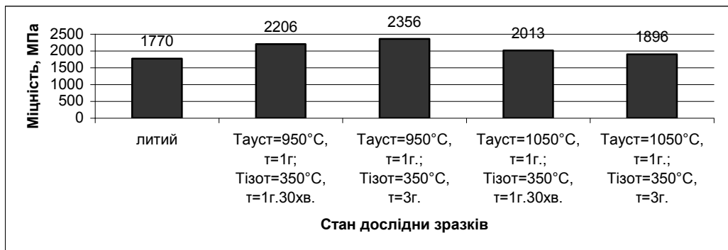
Рис. 7 Залежність межі міцності високохромистого чавуну від температури аустенізації та часу витримки при температурі 350°C
