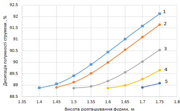
Рисунок 1 Залежність дисипації потужності струменя від висоти розташування фурми над рівнем спокійної ванни й витрати дутьтя.
