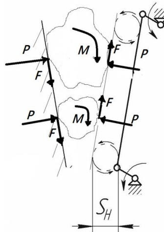
Рисунок 2 - Кінематична схема дробарки з паралельно-коловим рухом рухомої щокі до нерухомої
