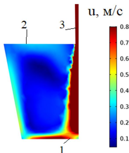
Рис. 2. Поля швидкостей потоків сталі в поперечному перерізі комплексу струмів металу - проміжний ківш:
