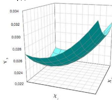
Рис. 2 Поверхня відгуку «абразивна твердість»
