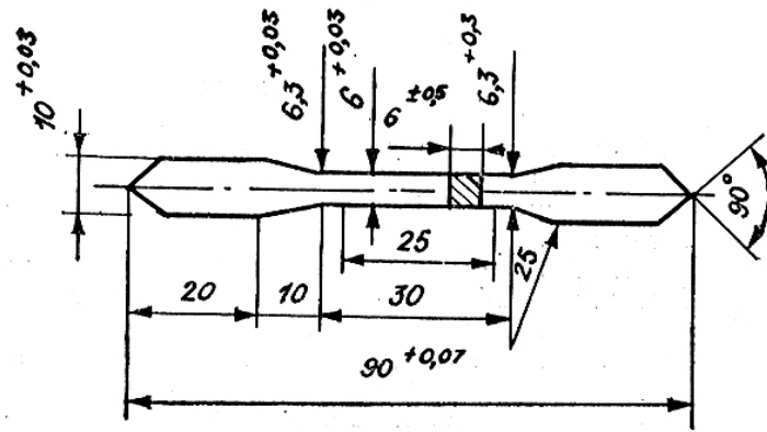
Рисунок 1 – Зразок для випробувань
