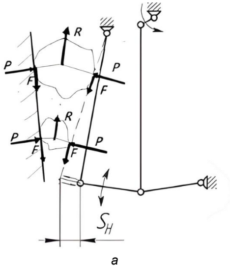
Рисунок 1 - Кінематичні схеми щоківних дробарок а – з простим рухом щоки; б – зі складним рухом щоки
